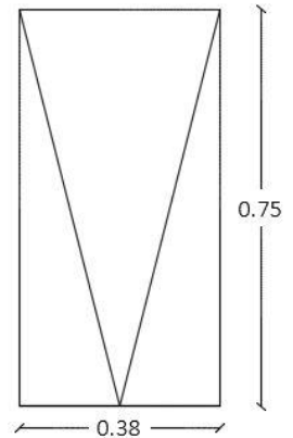
Plancha en lámina de hierro de 3/8" de espesor.
